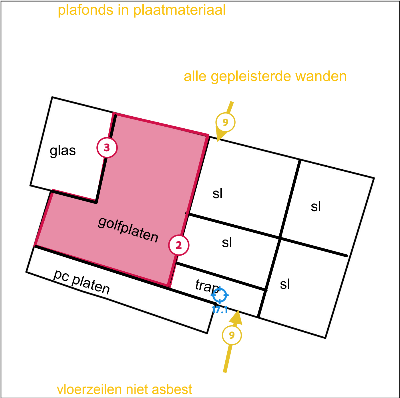
Legende van plan 1.2: Hoofdgebouw plan 1e
